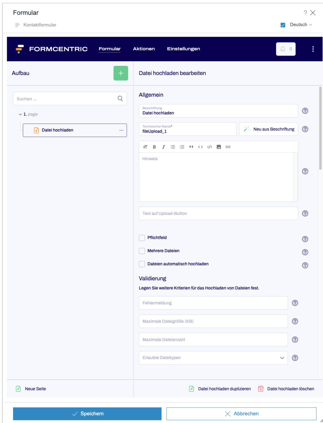
Abbildung 3.27. Datei hochladen
