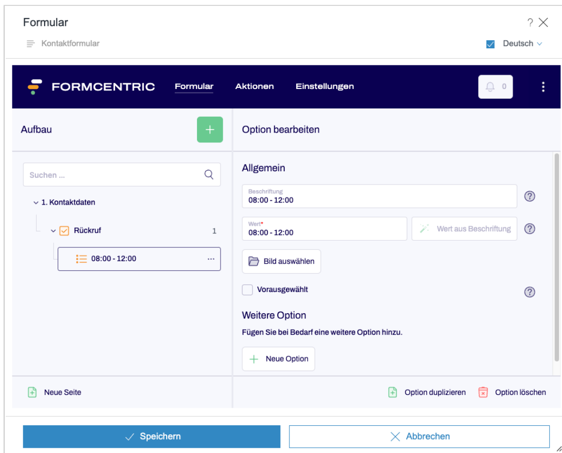
Abbildung 3.15. Option bearbeiten
