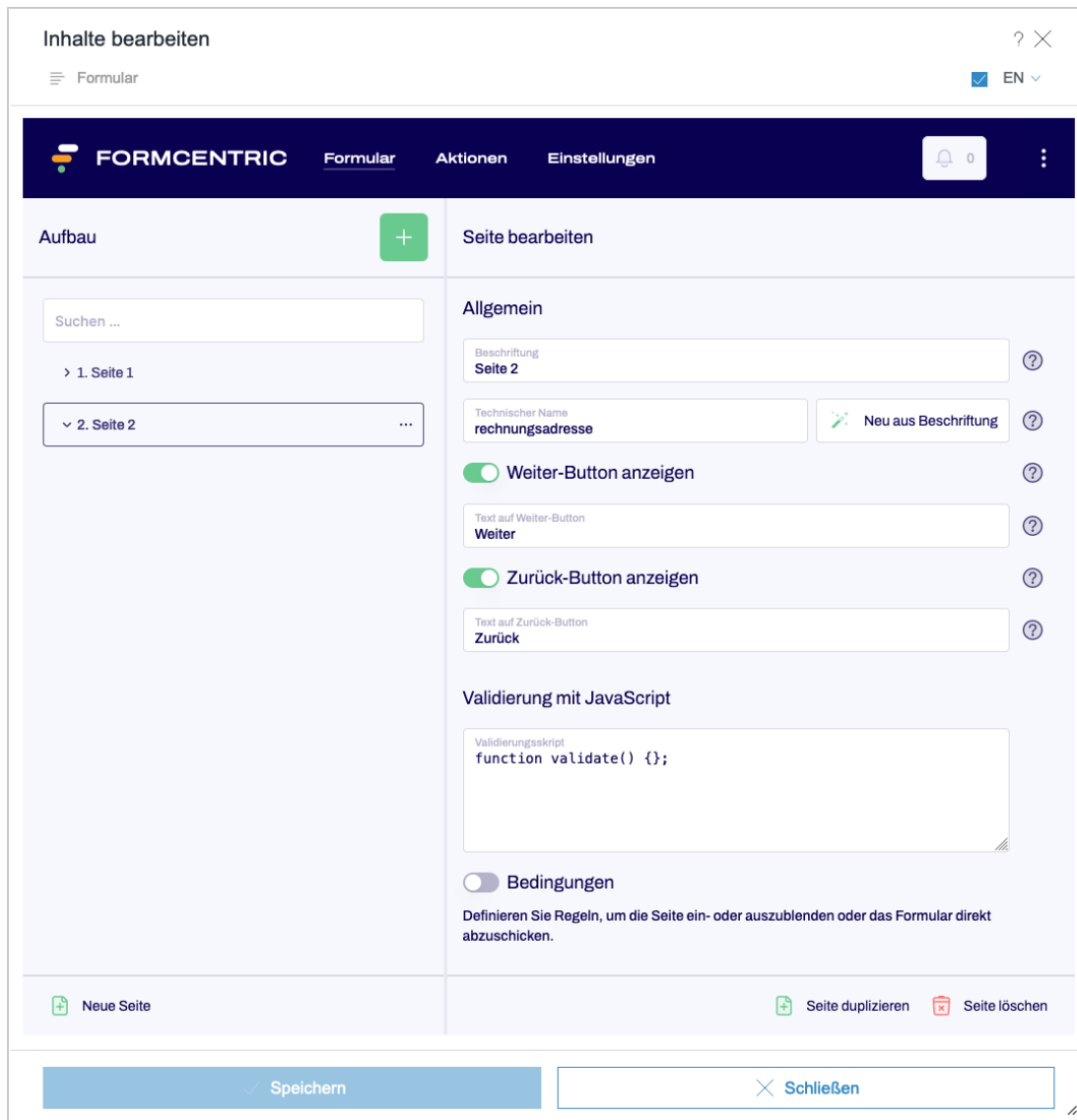
Abbildung 3.2. Seiteneigenschaften
