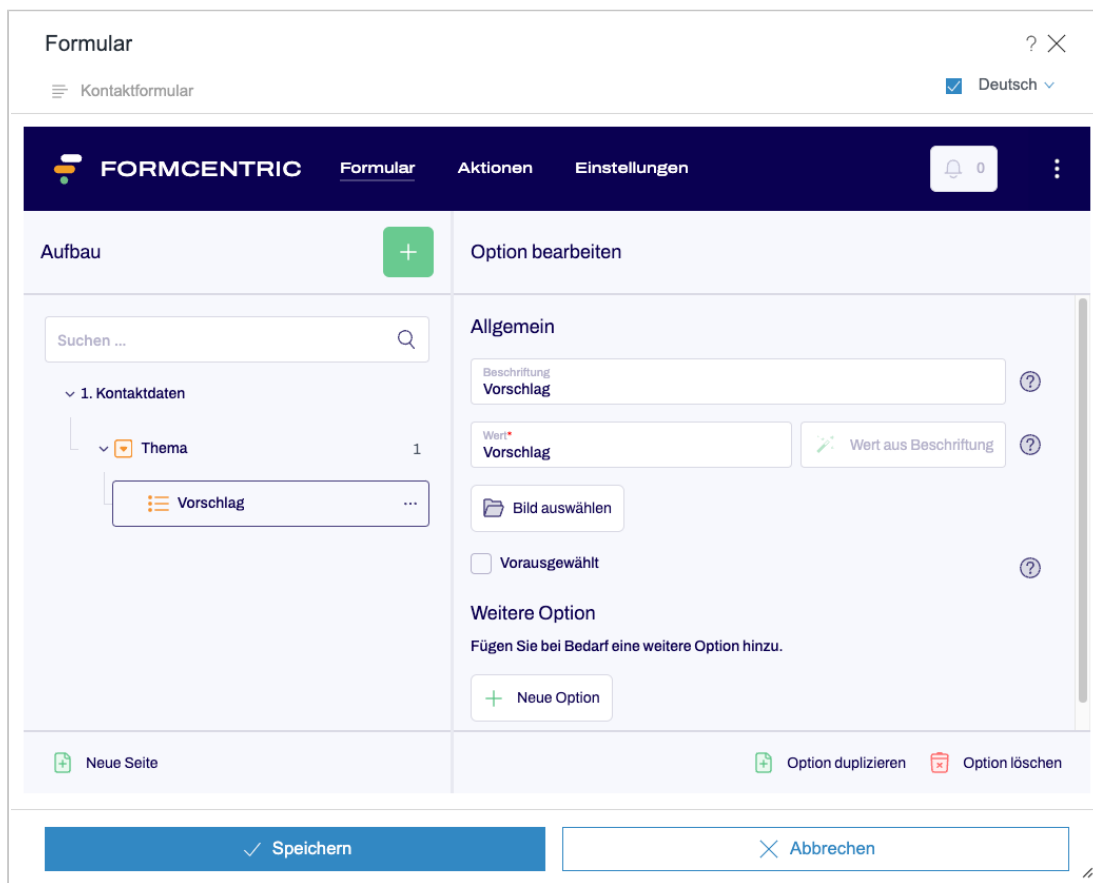
Abbildung 3.19. Option bearbeiten
