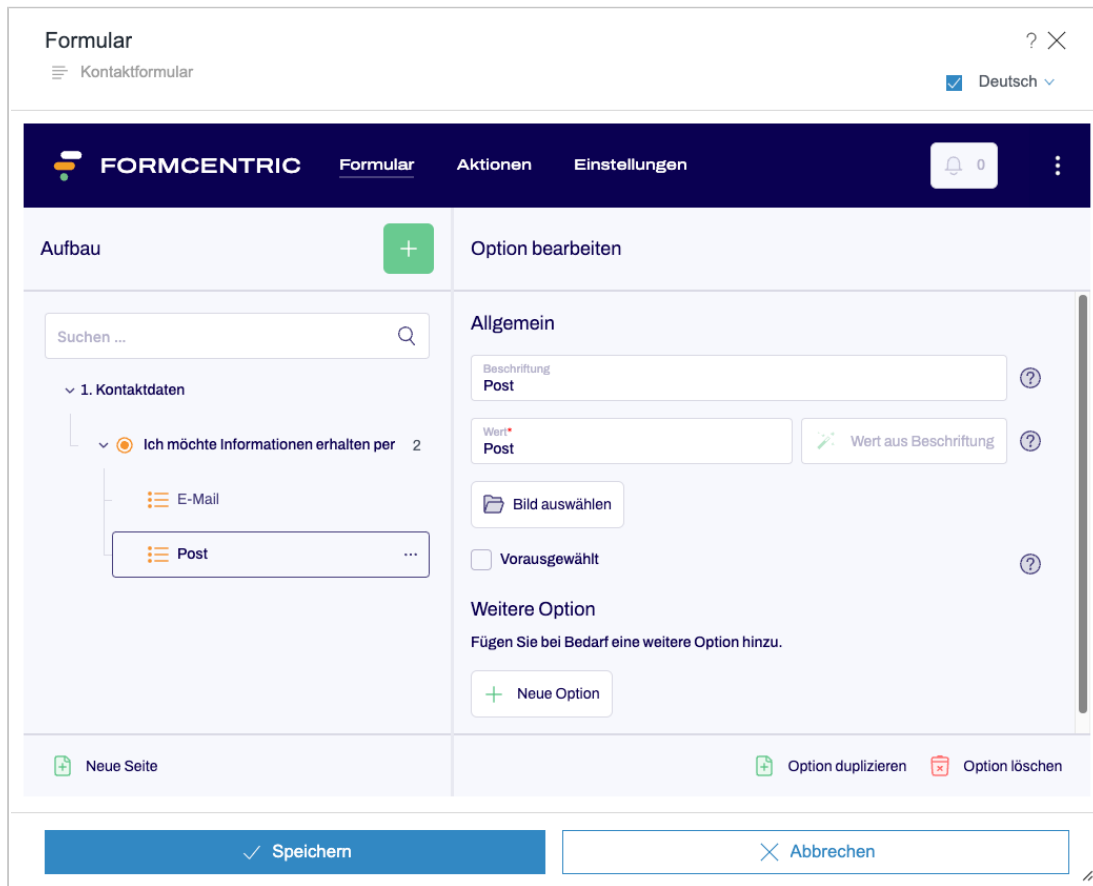
Abbildung 3.11. Option bearbeiten
