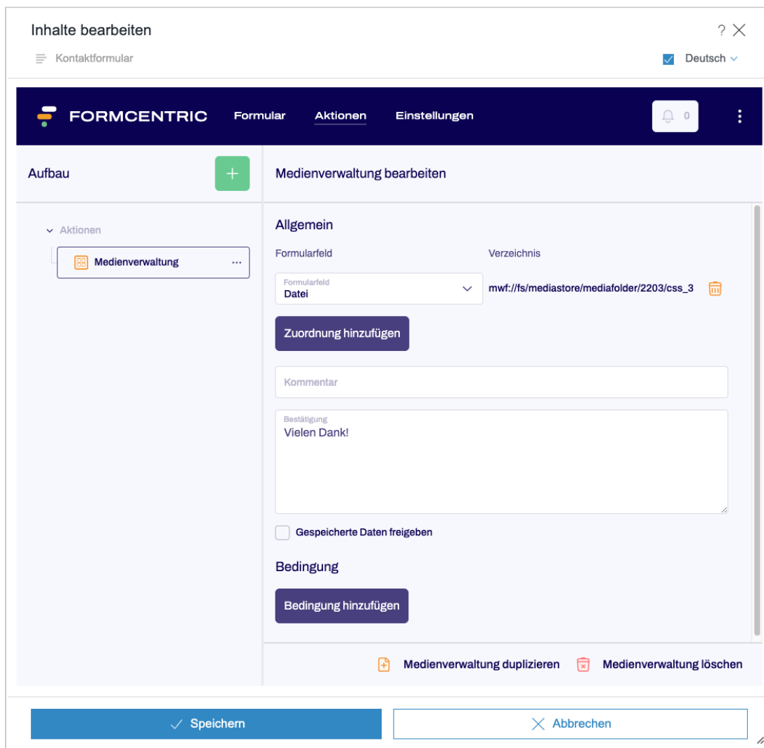
Abbildung 4.5. Medienverwaltung
