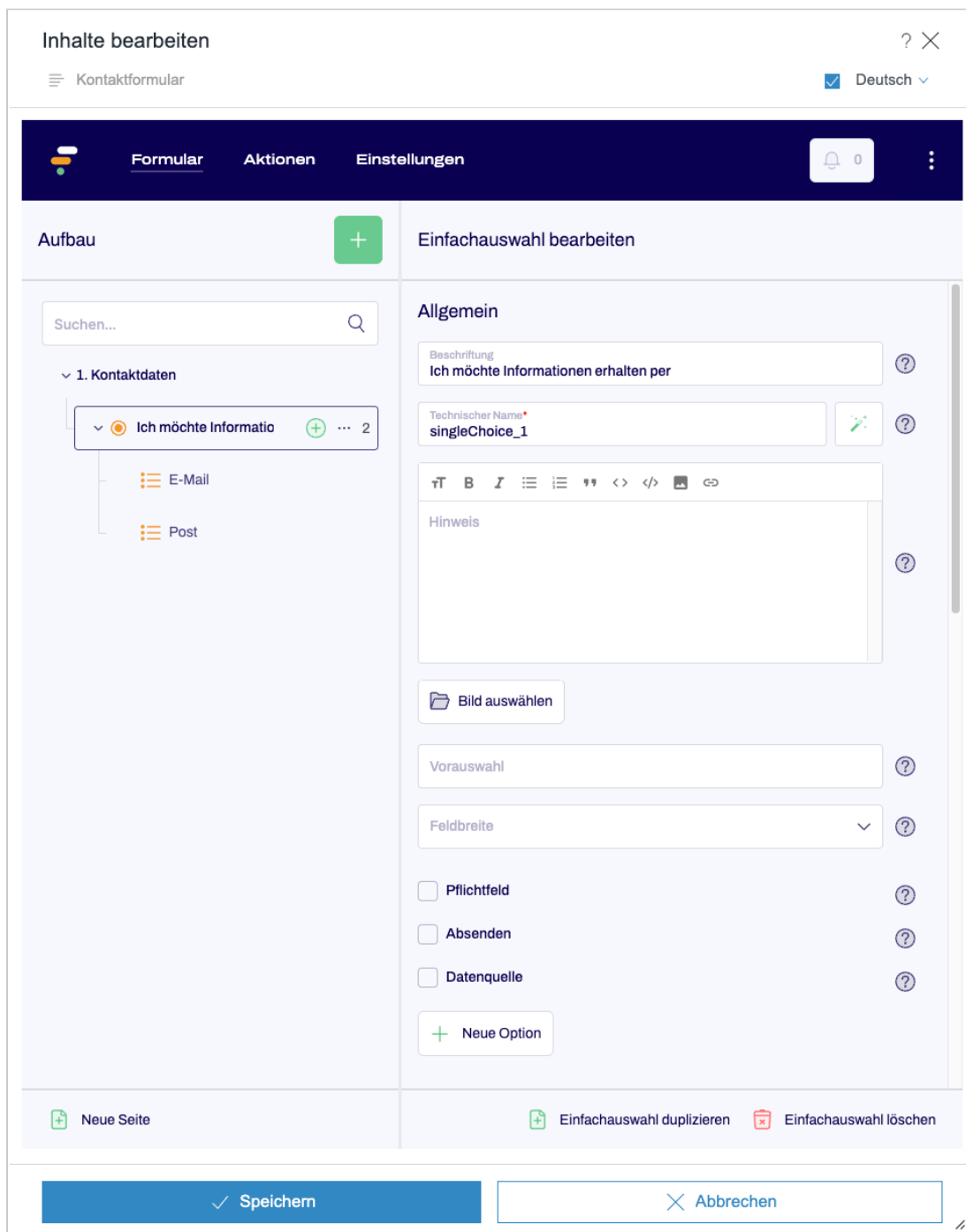
Abbildung 3.8. Einfachauswahl
