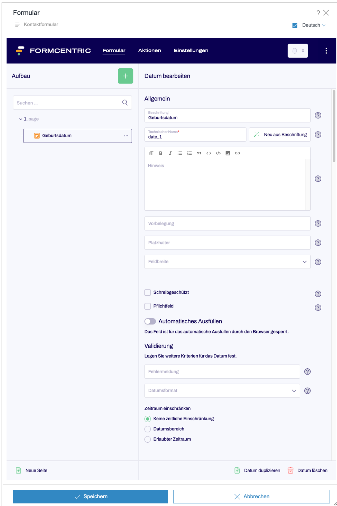
Abbildung 3.25. Datum
