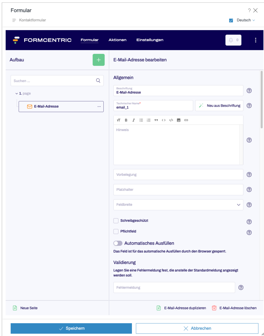
Abbildung 3.22. E-Mail
