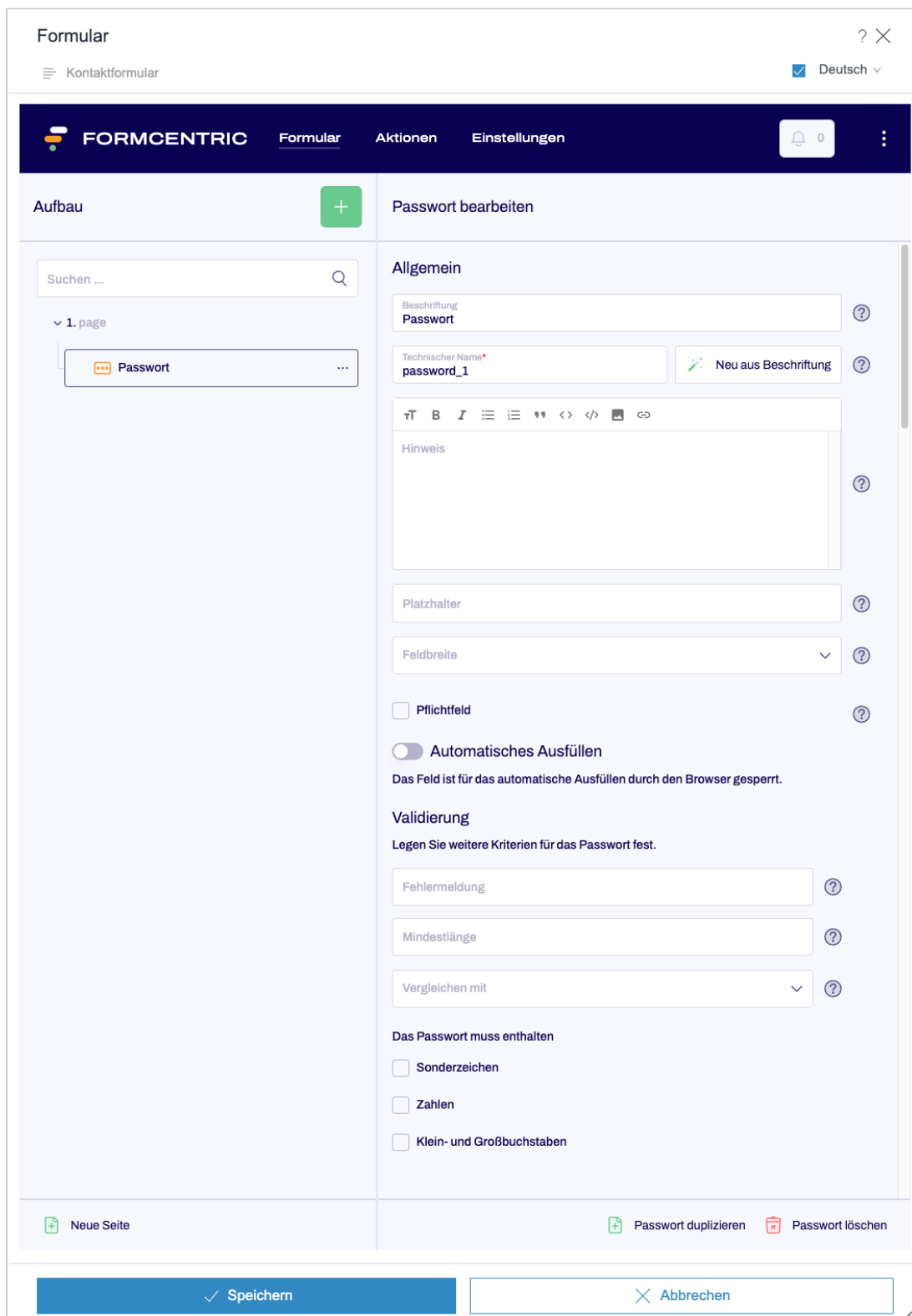
Abbildung 3.26. Passwort
