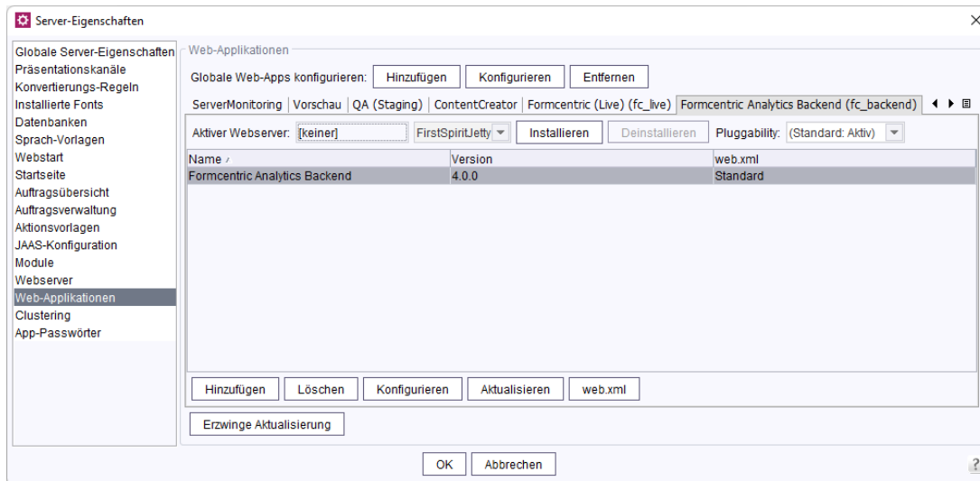
Abbildung 4.21. Globale Webapplikation mit installierter Web-Komponente
