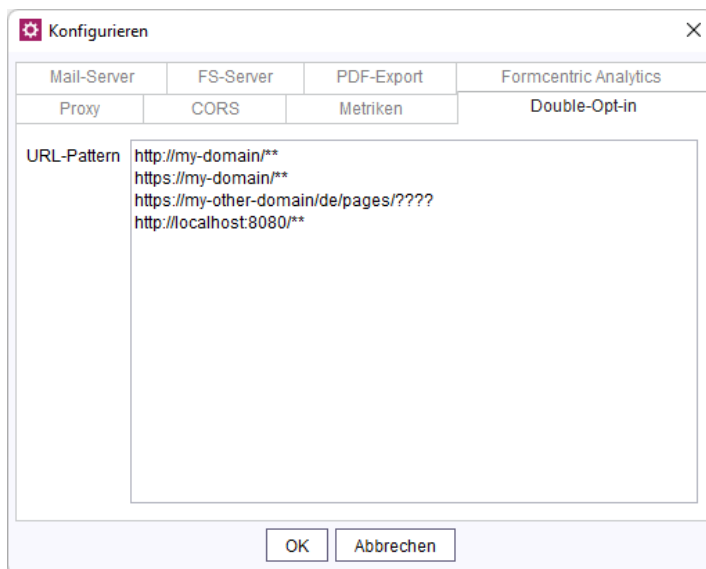
Abbildung 4.18. Konfiguration der URL-Pattern für das Double-opt-in
