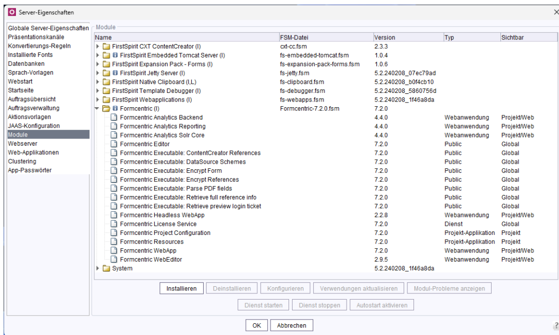
Abbildung 4.2. Liste der Module in den Server-Eigenschaften
