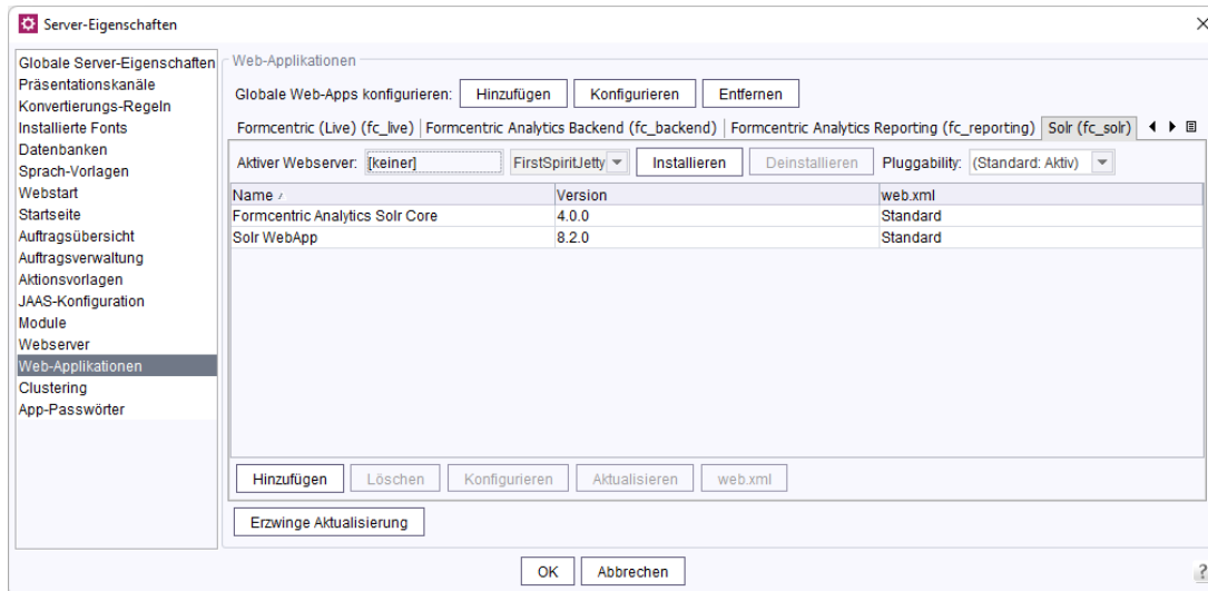
Abbildung 4.35. Solr-Webapplikation mit installierten Web-Komponenten
