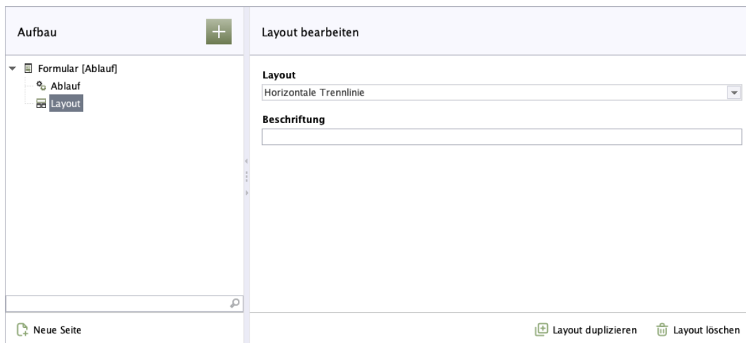
Abbildung 2.35. Layout
