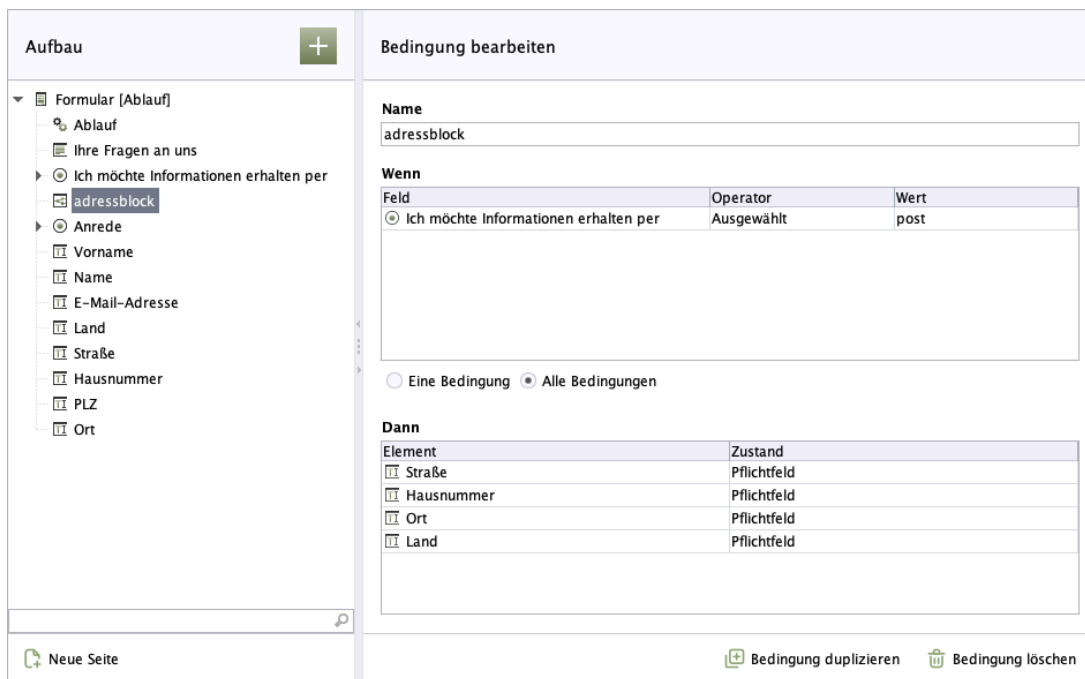
Abbildung 2.30. Bedingung
