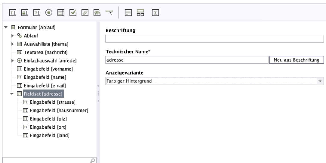
Abbildung 2.33. Fieldset
