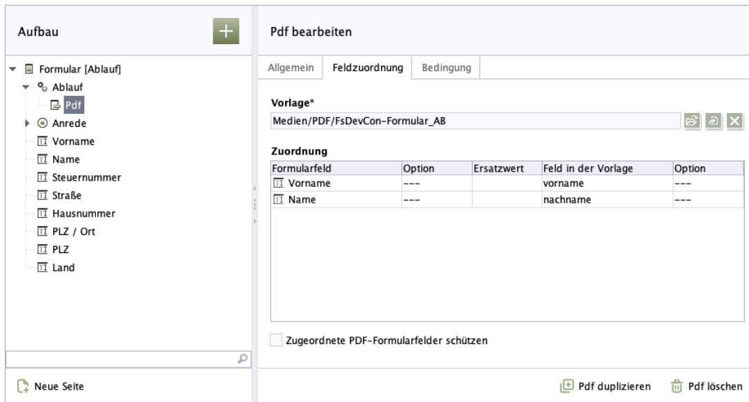
Abbildung 2.40. PDF
