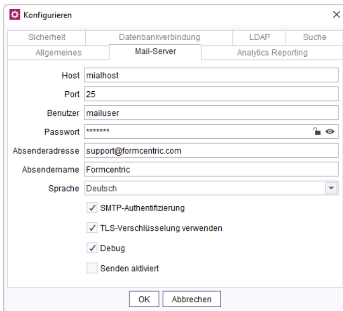
Abbildung 4.23. Konfiguration der Analytics-Backend-Webapplikation im Register „Mail-Server“
